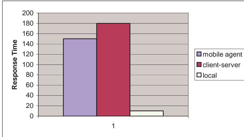
شکل ۶-۵- زمان پاسخ در حالتی که میزان استفاده از CPU، ۱۰۰٪ باشد.
